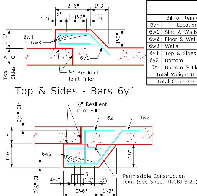
Bottom - Bars 6y2 & 6z
