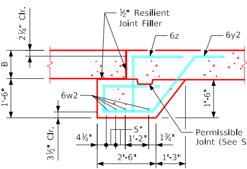
Bottom - Bars 6y2 & 6z
