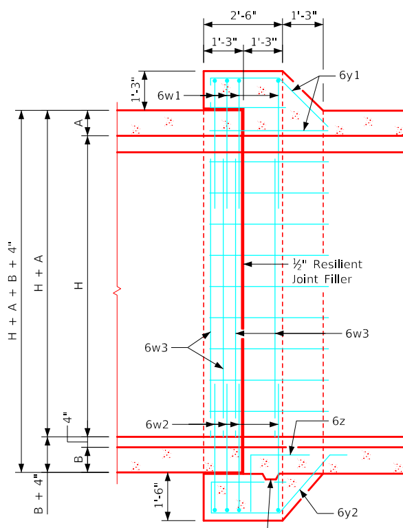
Longitudinal Section
