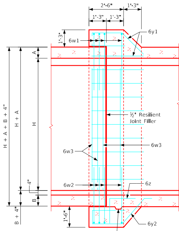
Longitudinal Section
